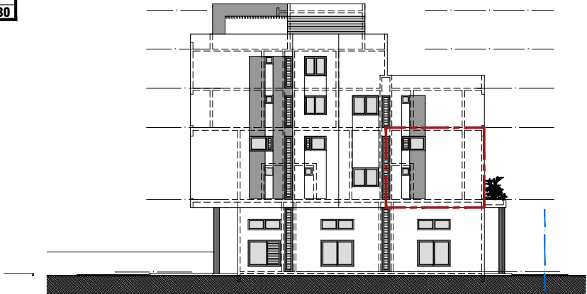
ELEVATION 1
